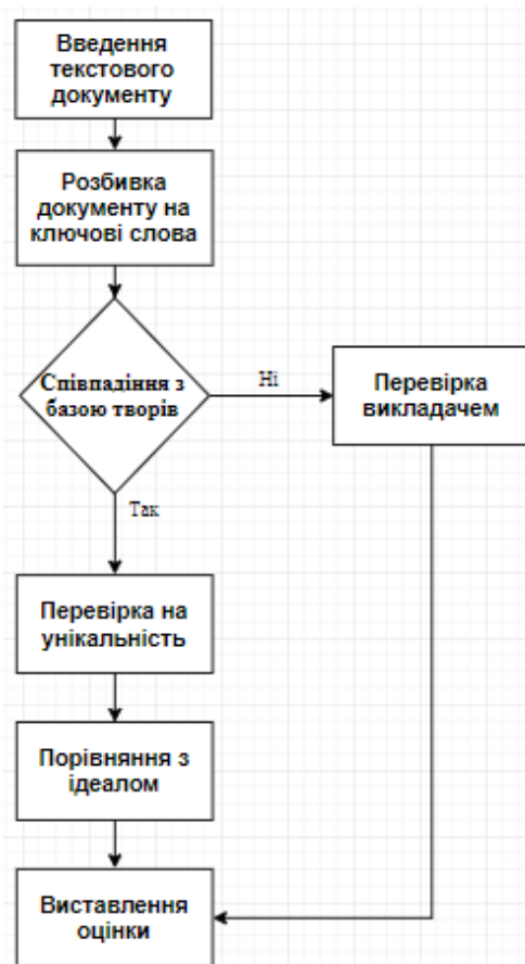
Рис. 1.1 Блок-схема дії програмного забезпечення для перевірки творів
