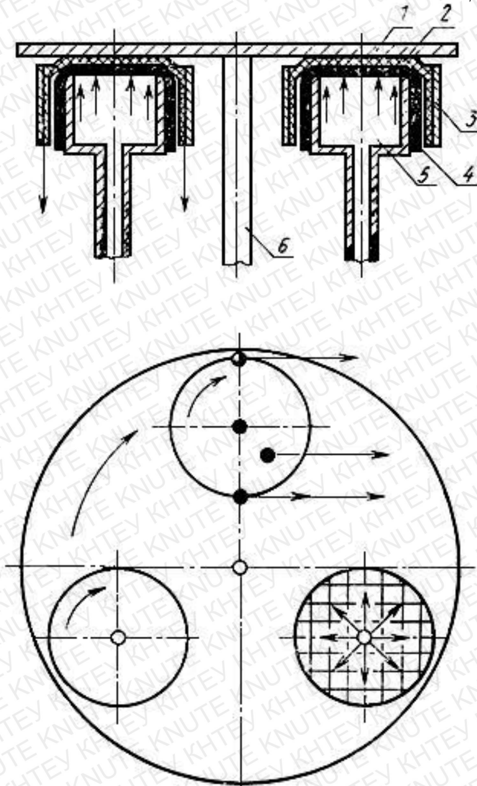
Рис. 1. Схематичне зображення приладу типу ТІ-1М для випробування тканин стійкості до стирання: 1 - стираючий диск; 2 - проба; 3 - обойма; 4 - мембрана; 5 - головка; 6 - вісь
