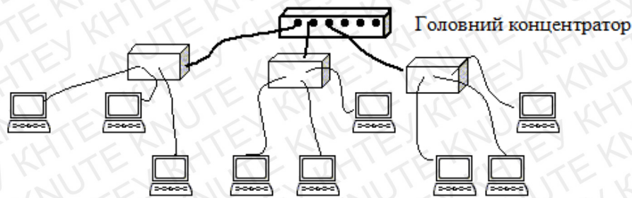
Рисунок 0.10. Топологія типу «зірка-кілеце»
