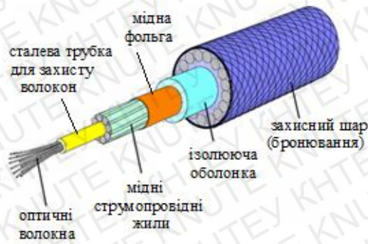
Рисунок 0.4. Волоконно-оптичний кабель
