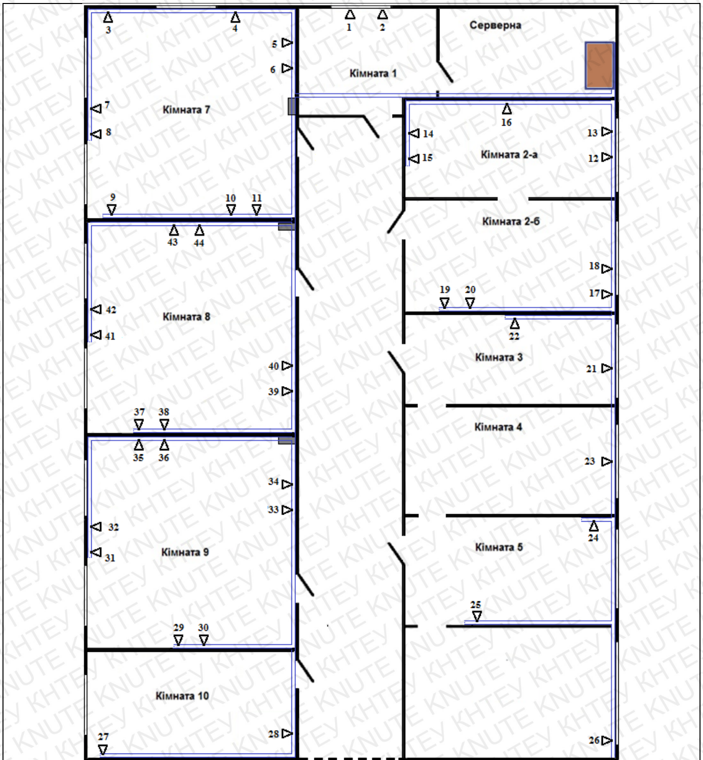
Рисунок 4. Схема розташування телекомунікаційних розеток
