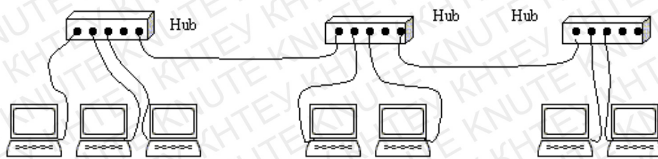
Рисунок 0.9. Топологія типу «зірка-шина»
