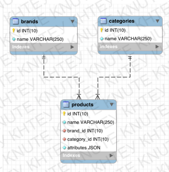
Рис.2.3. Приклад структури БД MySQL
