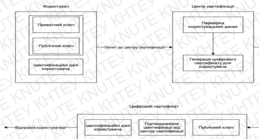
Рис. 1.2. Схема роботи центру сертифікації
