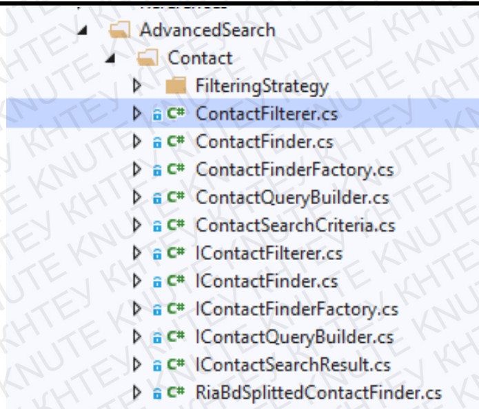
Рис. 3.7. Основні створені класи програмного модулю Advanced Search by Name
