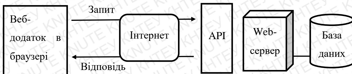
Рис. 2.1. Схема роботи API технологій
