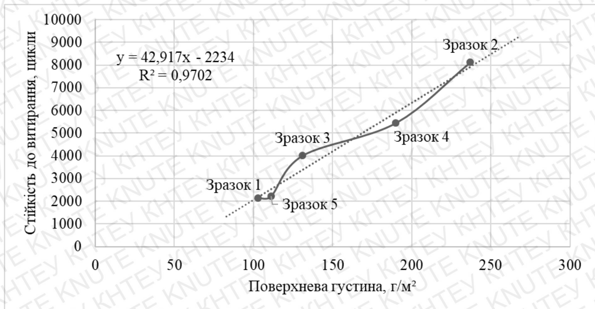
Рис.2.13. Графік залежності стійкості до витирання та поверхневої густини
