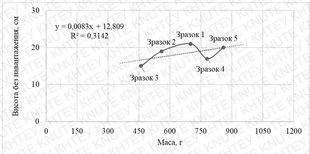
Рис. 2.12. Графік залежності маси та висоти без навантаження
